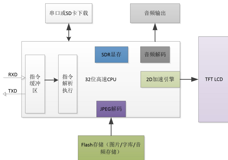
图 2-1 M 系列串口屏内部结构图
