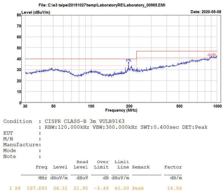
图 5-6 辐射测试水平方向
