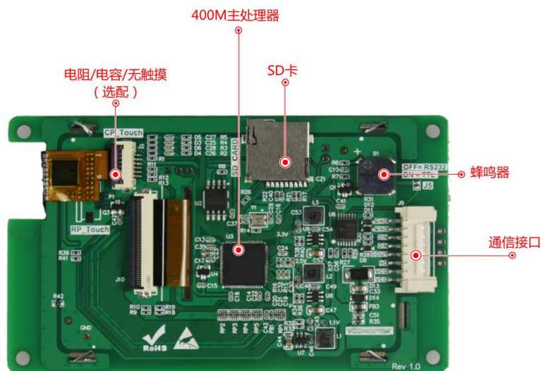
图 1-4 硬件配置图
