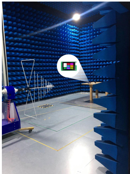
图 5-5 辐射测试图
