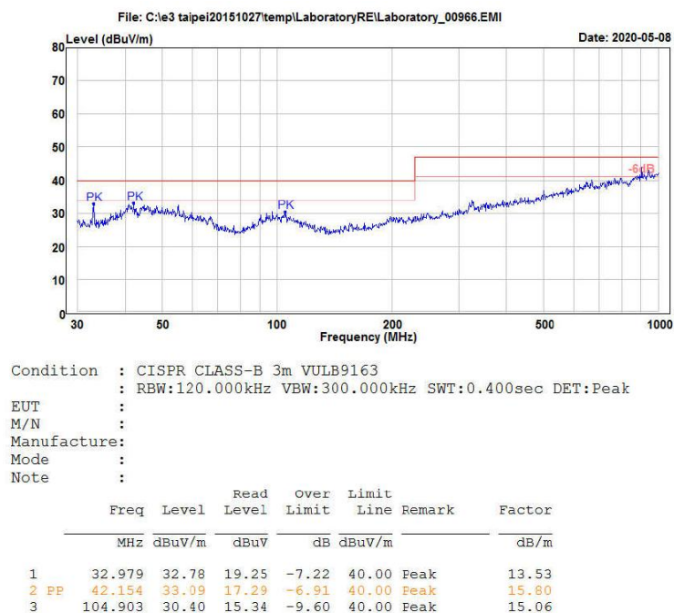
图 5-7 辐射测试垂直方向
